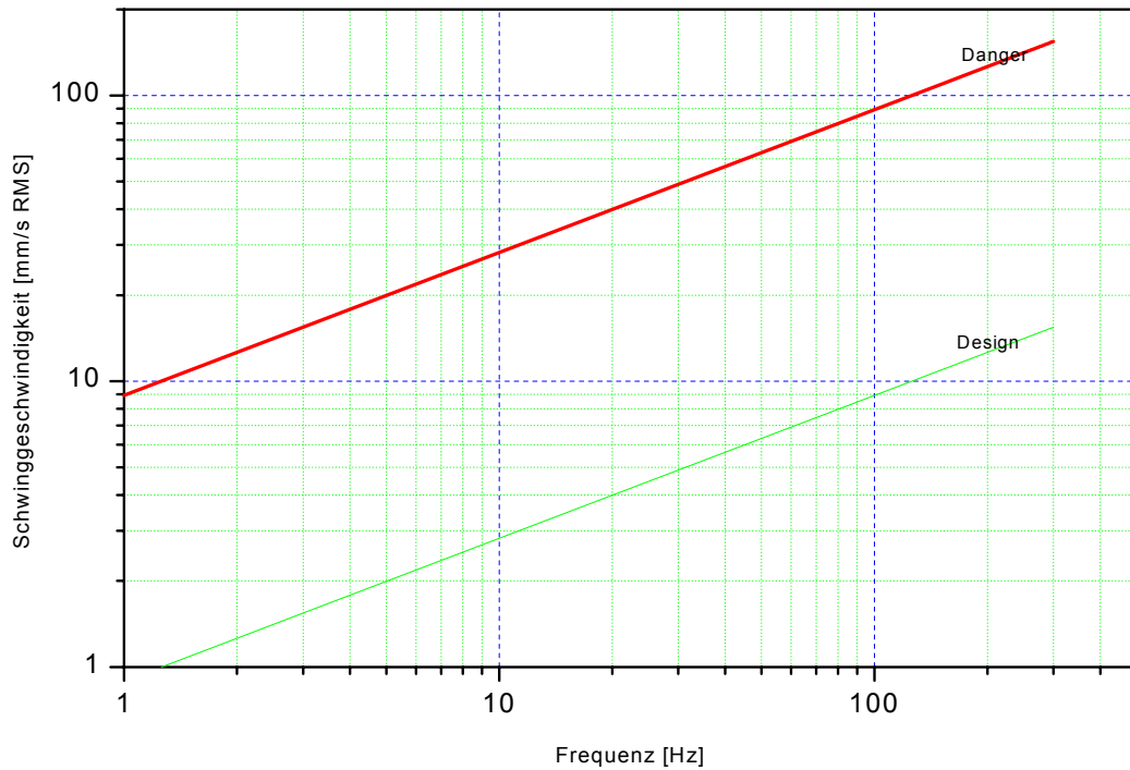
zulässige Schwinggeschwindigkeiten für Rohrleitungen in der petrochemischen Industrie nach Wachel/von Nimitz, bzw. TÜV
