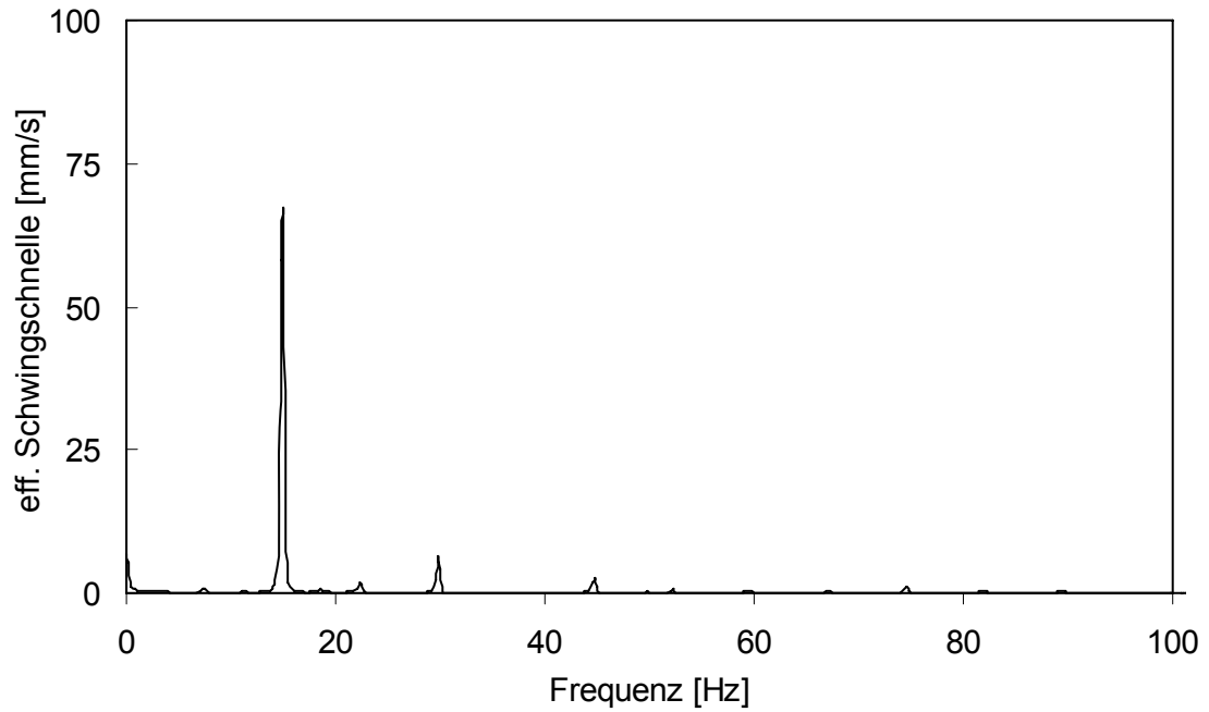
Abb. 6: Spektrum der Schwinggeschwindigkeit am Meßpunkt MP 10 in x-Richtung
