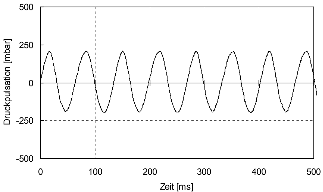
Abb. 4: Zeitverlauf der Druckpulsationen in der Saugleitung (1. Stufe)
