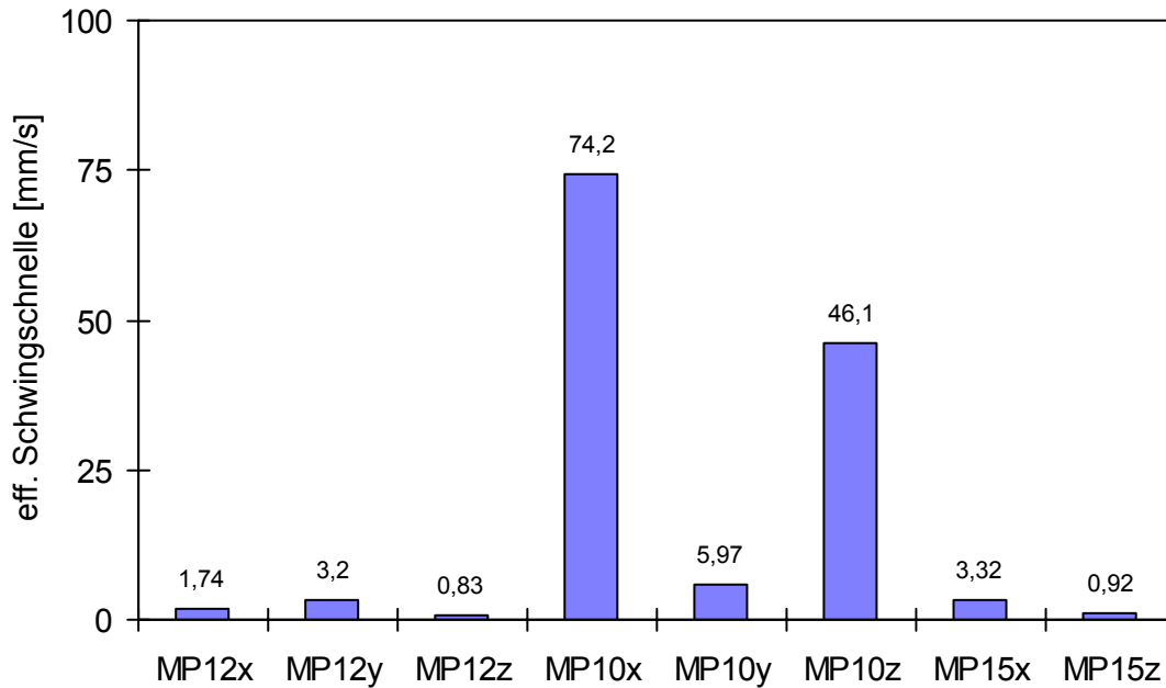
Abb. 5: Effektive Schwingschnelle auf der Rohrleitung an den unterschiedlichen Meßpunkten
