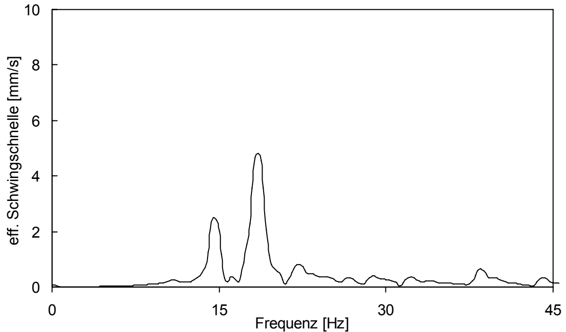
Abb. 7: Spektrum der Schwingschnelle an der Rohrleitung im Bereich des Meßpunktes 10 bei einer Impulsanregung und abgeschaltetem Kolbenverdichter
