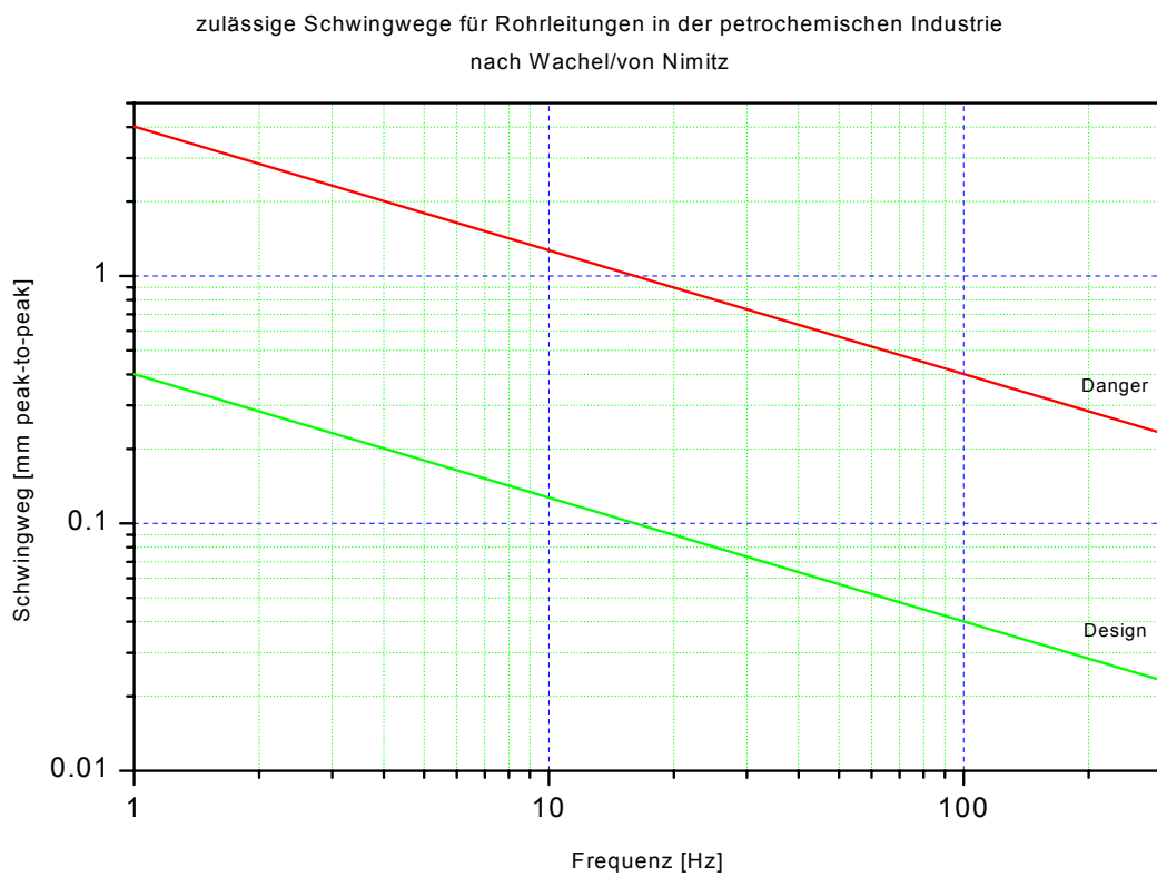
Abb. 3: Zulässiger Schwingweg als Funktion der Schwingfrequenz [4]
