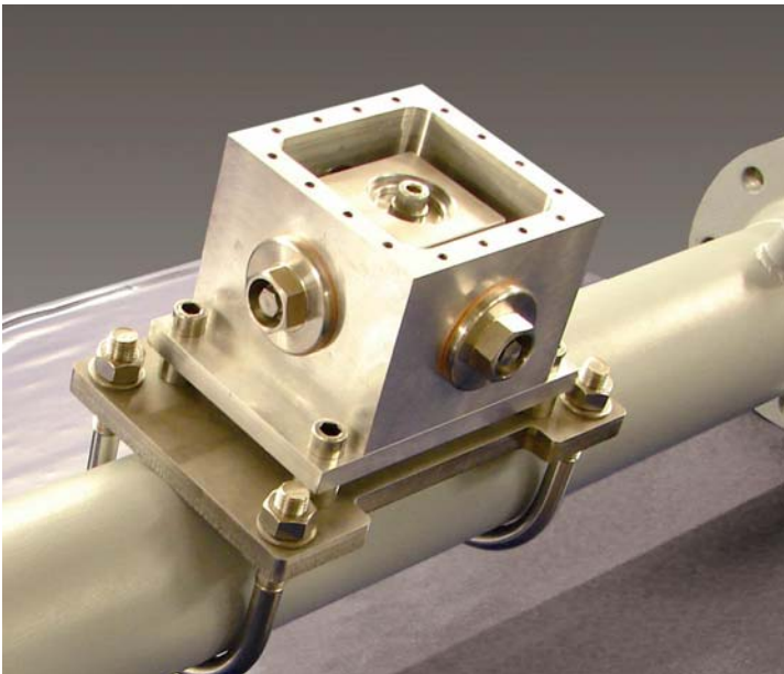
Typische Rohrleitungsbefestigung
