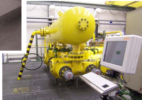
Referenzbeispiel an Kolbenverdichter
