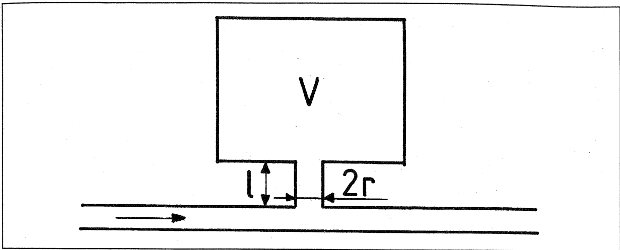
Bild 2: Helmholtz-Resonator (Reflexionsschalldämpfer)
