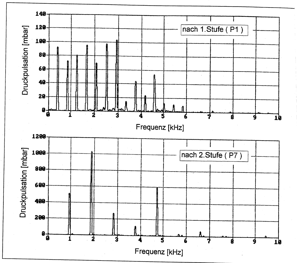
Bild 8: Amplitudenspektren der Druckpulsation nach der 1. Stufe (P1) und der 2. Stufe (P7) der Schraubenverdichteranlage im Ausgangszustand
