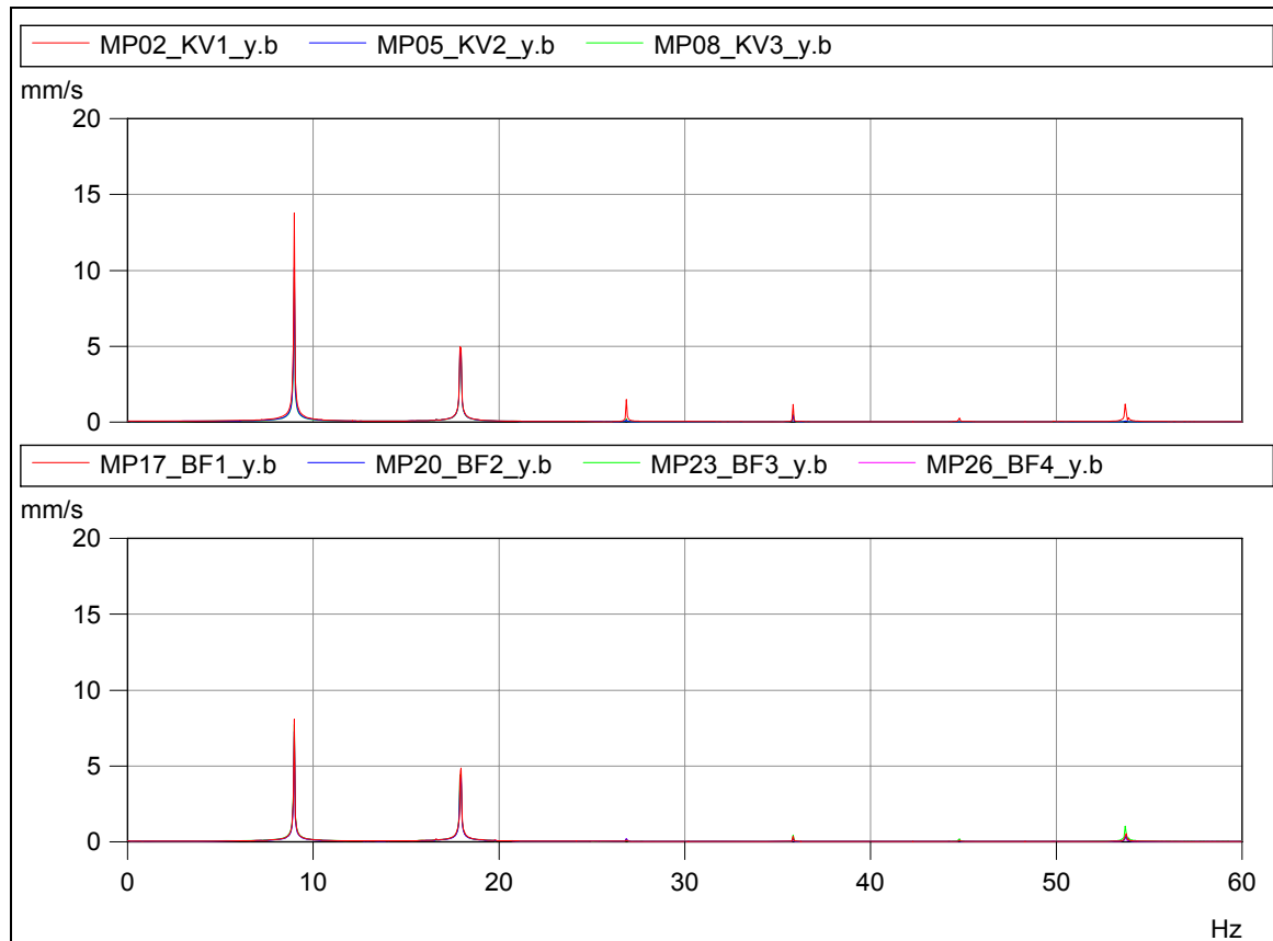
Abbildung 5: Amplitudenspektrum der gemessenen Verdichter- und Fundamentalschwingungen.
