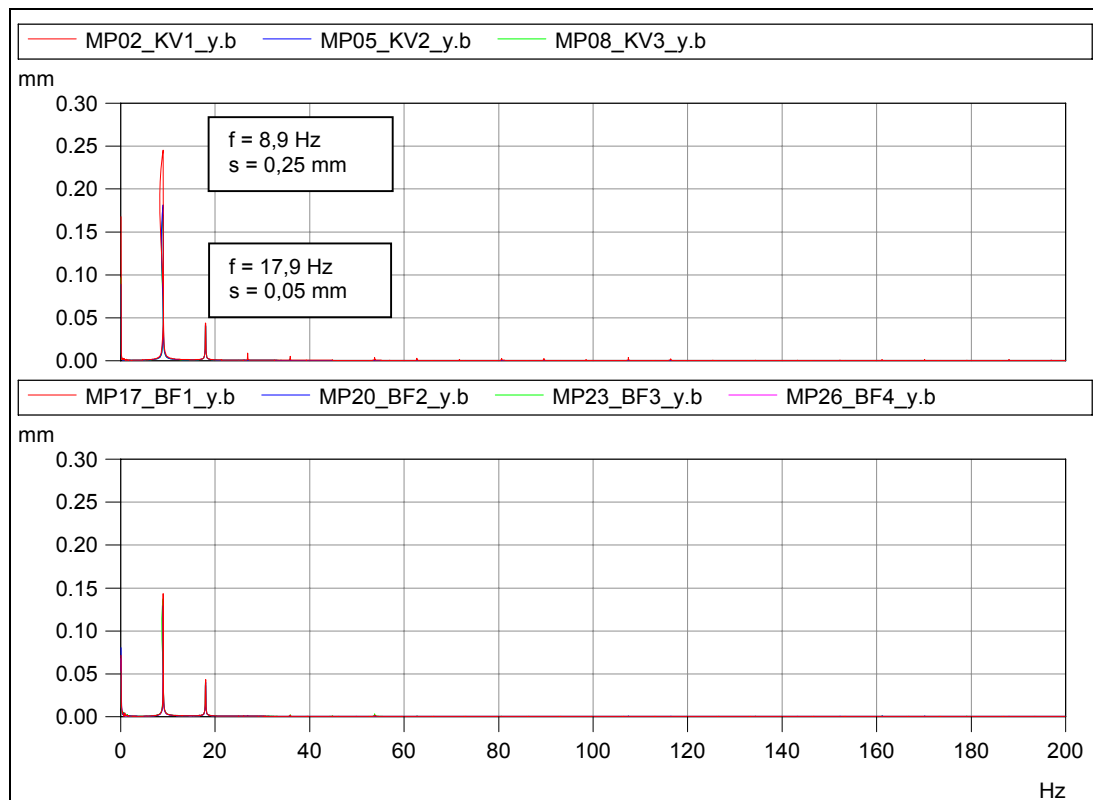
Abbildung 7: Amplitudenspektren der gemessenen bzw. integrierten Schwingwege am Verdichter und Fundament.
