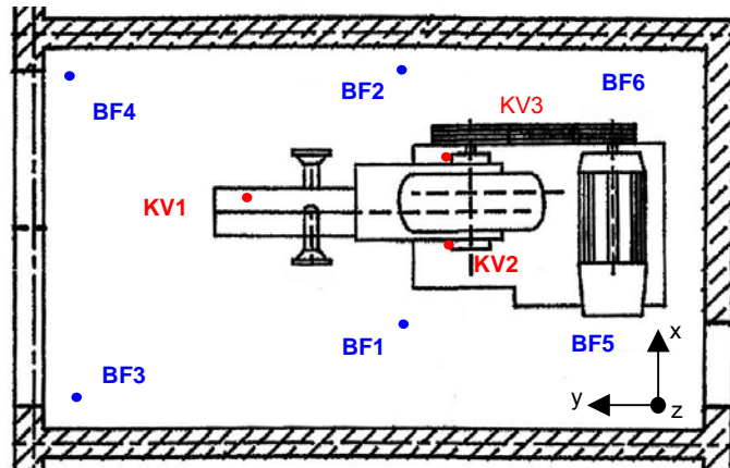
Abbildung 2: Lage der Messpunkte am Verdichter und Fundament.
