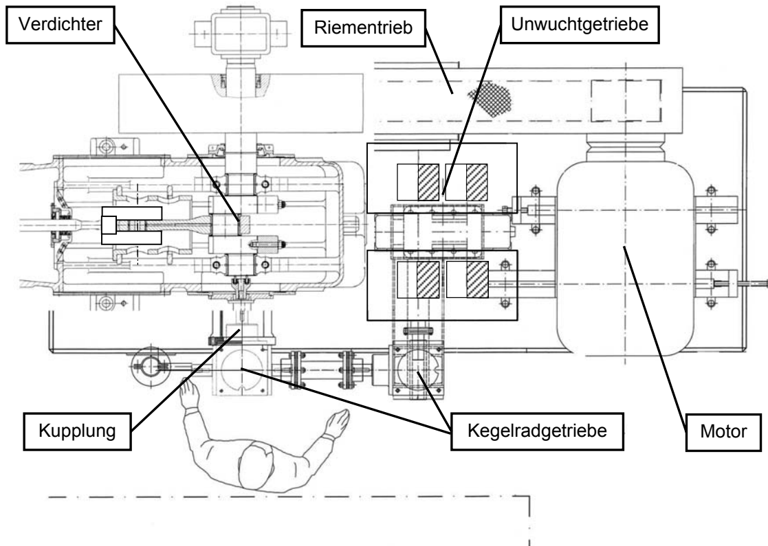
Abbildung 11 : Konstruktive Detailausführung der Minderungsmaßnahme Unwuchtgetriebe zwischen Kolbenverdichter und Antriebsmotor.
