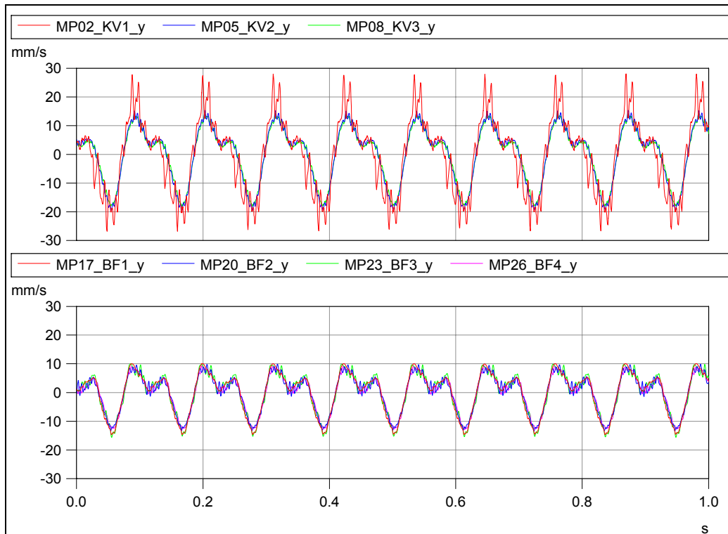
Abbildung 4: Zeitverlauf der gemessenen Schwinggeschwindigkeit am Verdichter und Fundament.
