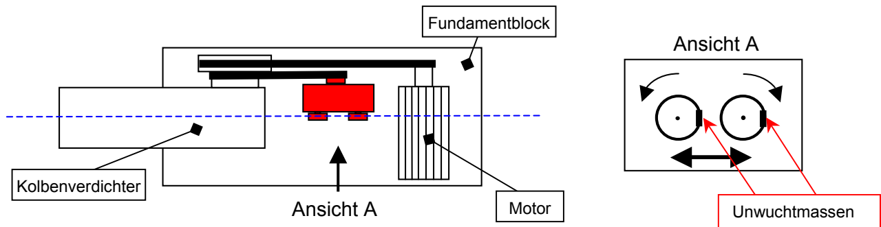
Abbildung 10: Prinzipskizze zur Montageposition des Unwuchtgetriebes zwischen Kolbenverdichter und Motor (links) sowie prinzipielle Anordnung der Unwuchtmassen und Drehrichtungen am Unwuchtgetriebe (rechts).
